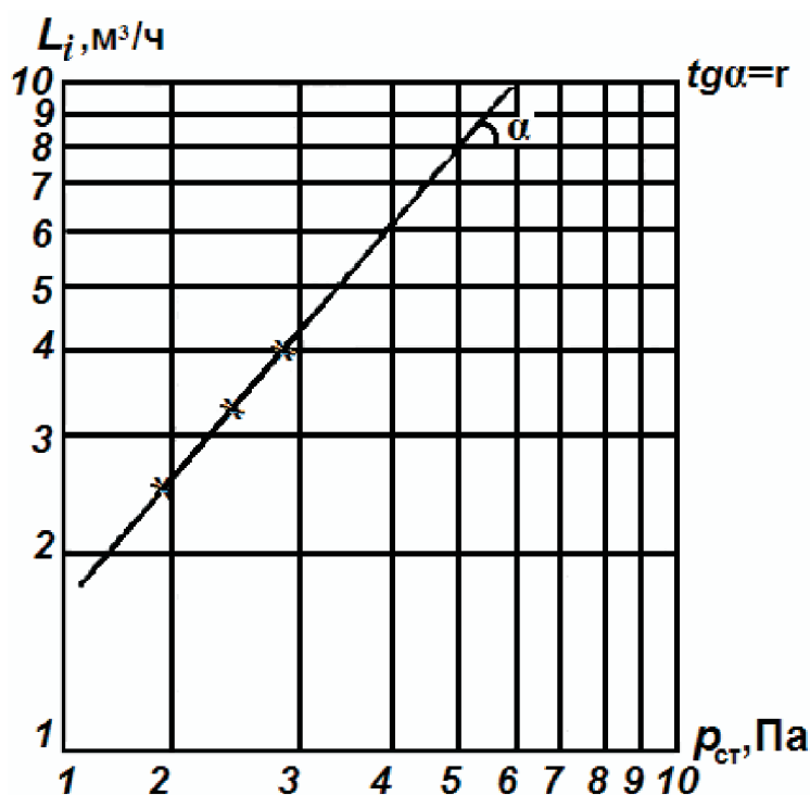
Рисунок 9.2 – График зависимости L_i = R (p_{стi})^r , полученный по результатам испытаний сетей воздуховодов на герметичность, где R – коэффициент градуировки, равный расходу воздуха при p_{ст} = 1 Па
